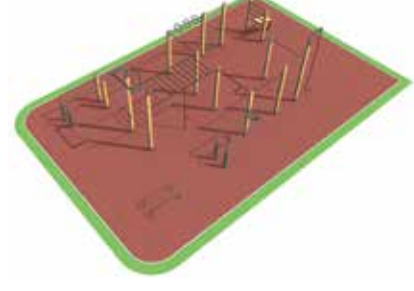
Larix Line XL 14 x 9,3 x 3,6m ΧΩΡΟΣ ΑΣΦΑΛΕΙΑΣ: 15,2 x 9,6m (145,9m 2 )
