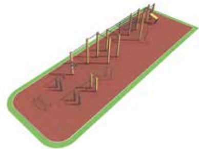
Larix Line L 14,5 x 3,4 x 3,6m ΧΩΡΟΣ ΑΣΦΑΛΕΙΑΣ: 19,6 x 6m (117,6m 2 )
