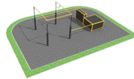
SIMPLE XS 5,6x2,7m / ΧΩΡΟΣ ΑΣΦΑΛΕΙΑΣ: 9,2x6,5m
