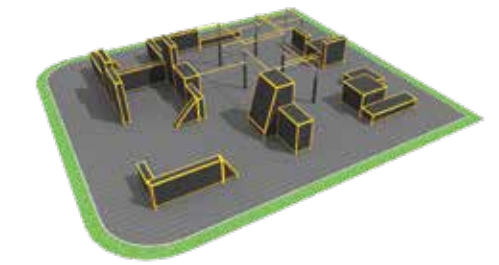
SIMPLE XL 11,8x10,2m / ΧΩΡΟΣ ΑΣΦΑΛΕΙΑΣ: 14,9x13,3m
