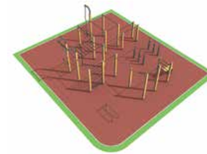
Larix STANDARD XL 7,2 x 7,2 x 3,6m ΧΩΡΟΣ ΑΣΦΑΛΕΙΑΣ: 12,7 x 11,2m (142,24m 2 )
